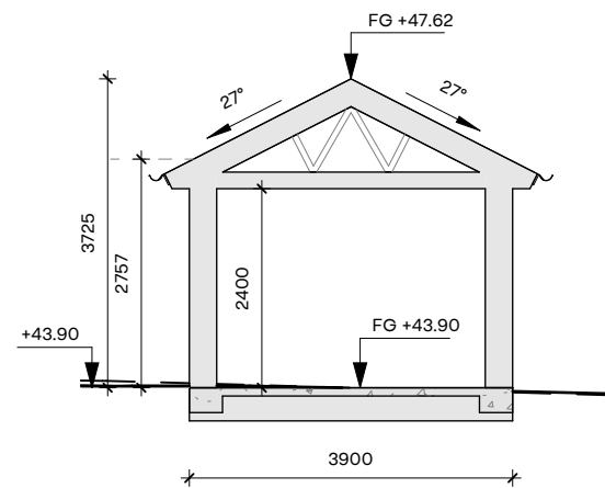
C SEKTION C-C 1:100
