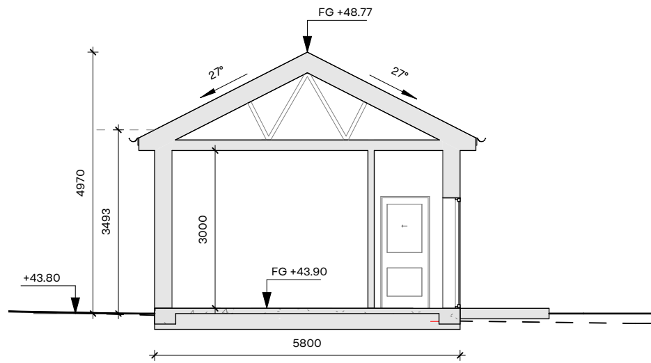
B SEKTION B-B 1:100
