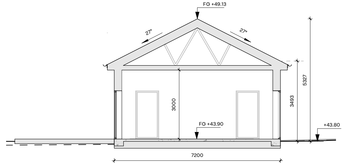
A SEKTION A-A 1:100
