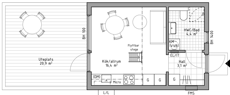
Entréplan
